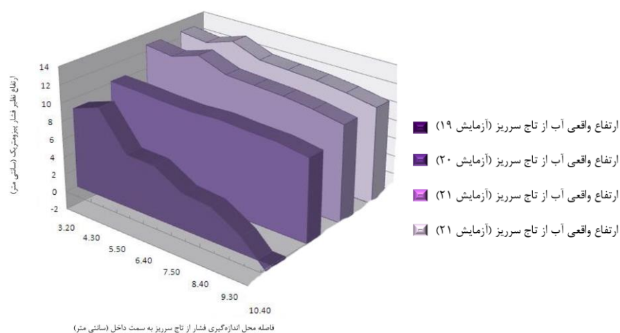
شکل ۱۱: نمودار تغییرات فشار در بدنه سرریز شاهد با آرایش شش گرداب شکن و ارتفاع ۵/۲ سانتی‌متر و ضخامت ۹ میلی‌متر
