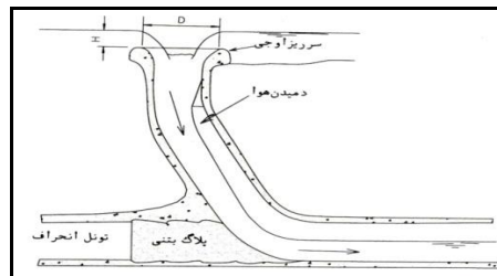
شکل ۱: نمایش یک سرریز نیلوفری
