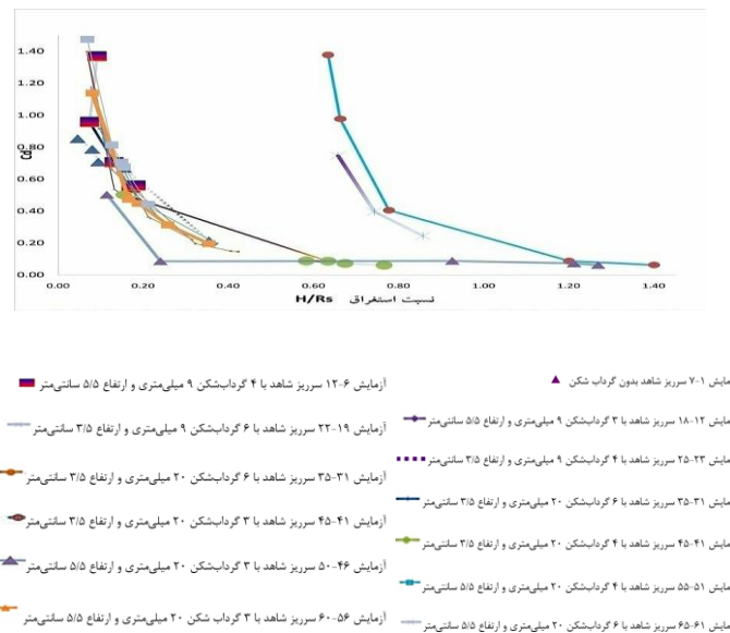
شکل ۱۲: نسبت استقرای به ضریب تخلیه در مجموعه آزمایش‌های مربوط به سرریز شاهد با و بدون استفاده از گرداب‌شکن
