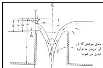
شکل ۲: مقطع یک سرریز نیلوفری
