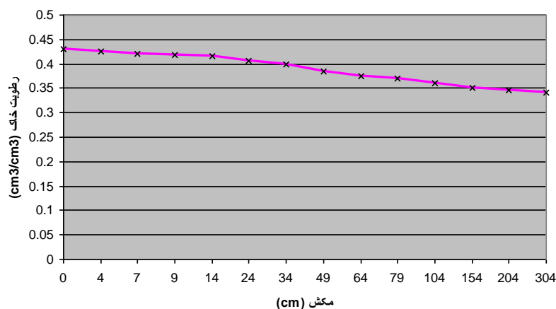
شکل ۱: منحنی مشخصه رطوبتی خاک طرح
