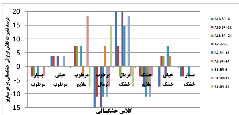
شکل ۵: درصد تغییر وضعیت فراوانی خشکسالی ها نسبت به دوره دیده بانی با توجه به دسته SPI در هر سناریو (۲۰۹۹-۲۰۸۰)
