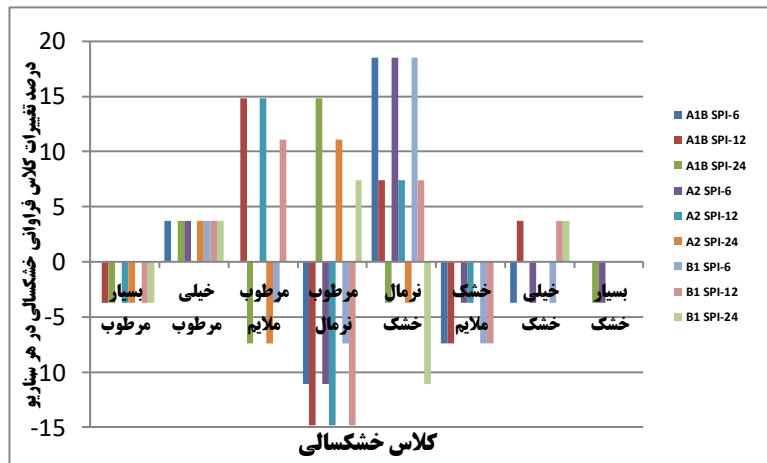
شکل ۴: درصد تغییر وضعیت فراوانی خشکسالی ها نسبت به دوره دیده بانی با توجه به دسته SPI در هر سناریو (۲۰۶۰-۲۰۴۶)
